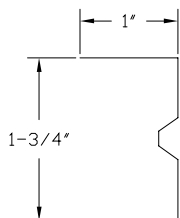
90° Edge Used on DE-90 DEA-90 & DEA 905
