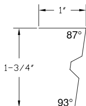
87°/93° Edge Used on DE,DEA,DEA-5 DE-DE,DEA-DE & DEA-DE-5
